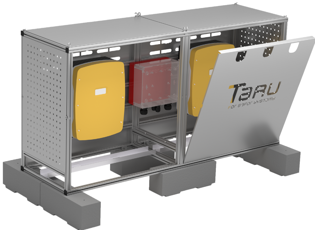
Wechselrichterunterstand L Basis + Erweiterung auf Betonsockel Inverter Shelter L Basic + Extension on Concrete Blocks
